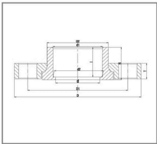
双片式法兰 PVC-C --ANSI Two-piece Flange PVC-C --ANSI
