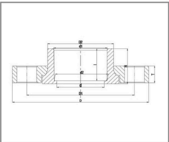
双片式法兰 PVC-U --ANSI Two-piece Flange PVC-U --ANSI
