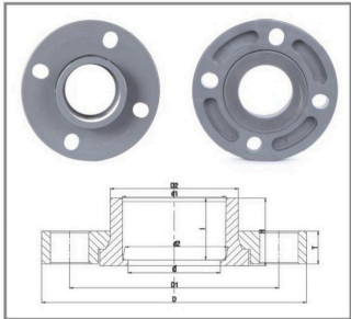
双片式法兰 PVDF --DIN Two-piece Flange PVDF --DIN
