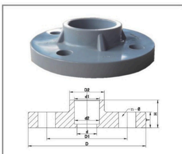
单片式法兰PVDF--DIN One-piece Flange PVDF--DIN
