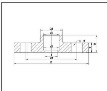
单片式法兰 PVC-C --JIS One-piece Flange PVC-C --JIS
