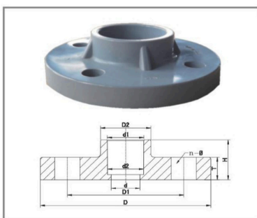
单片式法兰 PP-H --DIN One-piece Flange PP-H --DIN
